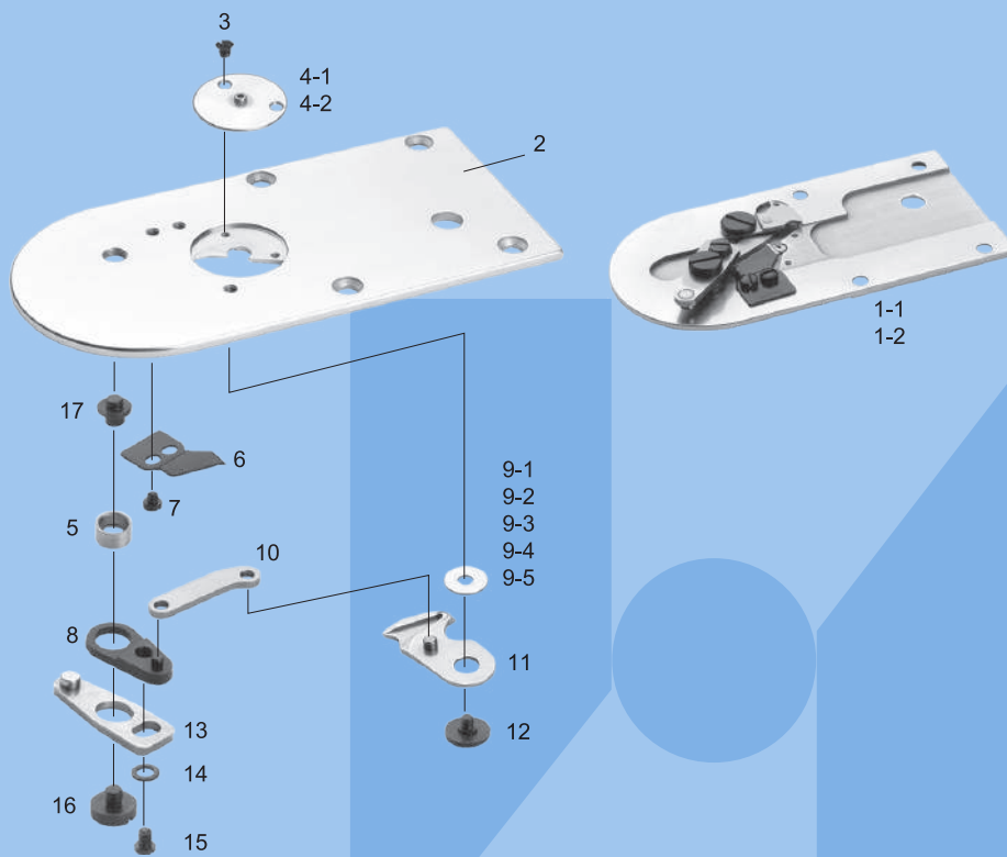
LK-1903A 剪线组件 ASSEMBLY FOR LK-1903A
