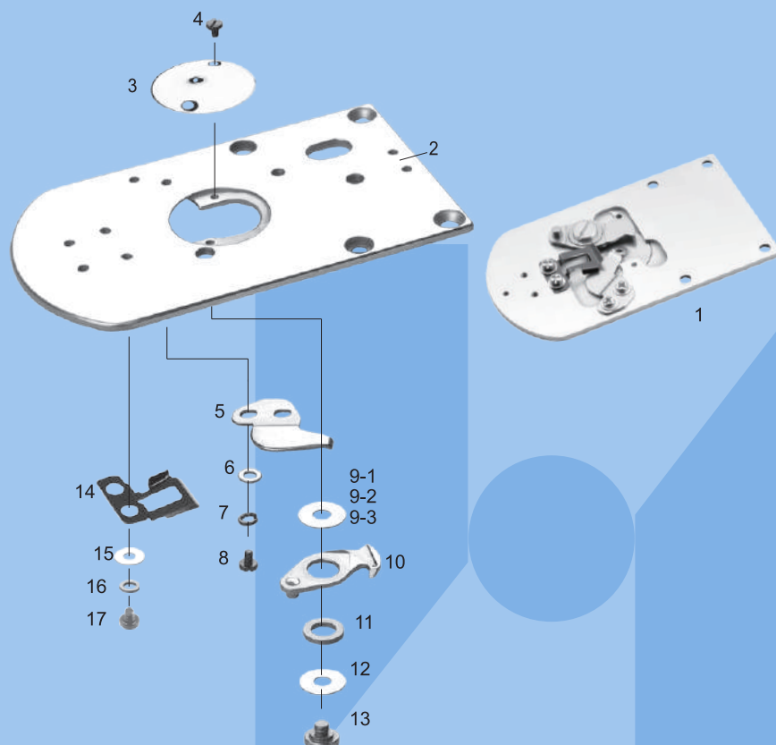
BE-438F 剪线组件 ASSEMBLY FOR BE-438F
